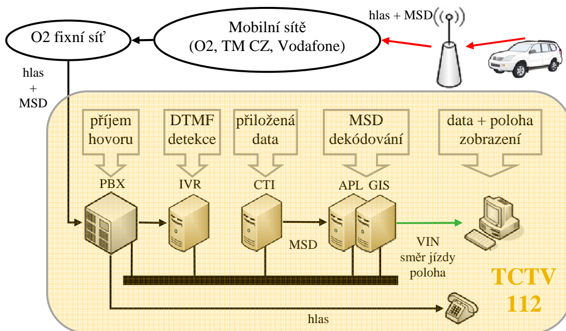
Obr. 13 Průběh eCall volání [43,44]
