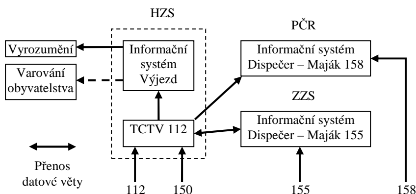
Obr. 3 Architektura informačního systému IZS [17]
