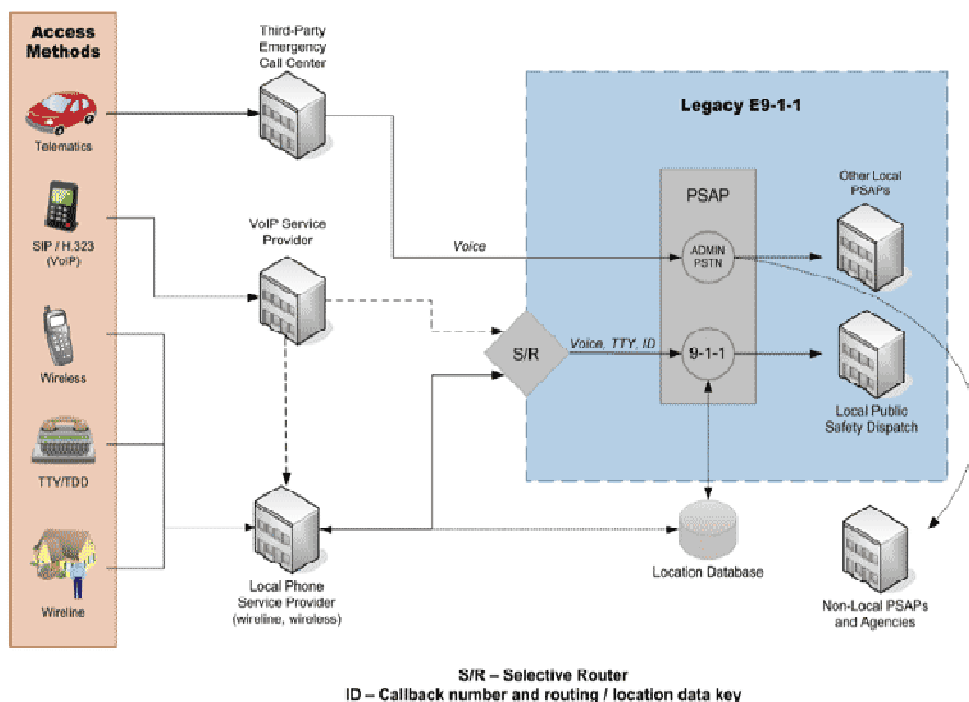
Obr. 27 Blokové schéma systému E911 [80]
