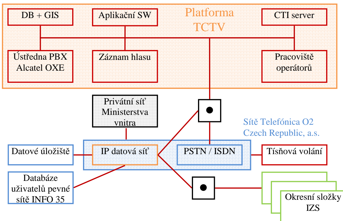
Obr. 6 Řešení systém komunikace TCTV 112 od NextiraOne Czech [33]
