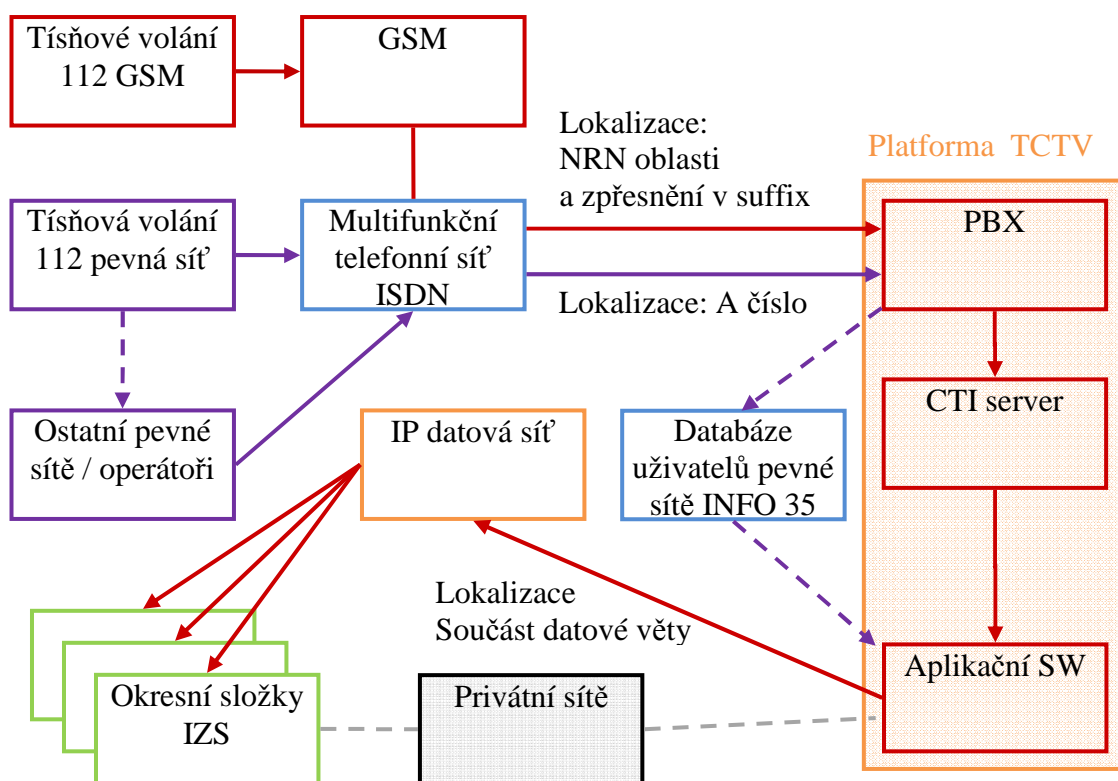
Obr. 10 Systém předávání informace o poloze volajícího [33]
