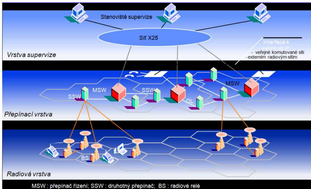
Obr. 4 Vrstvy infrastruktury sítě Pegas [25]
