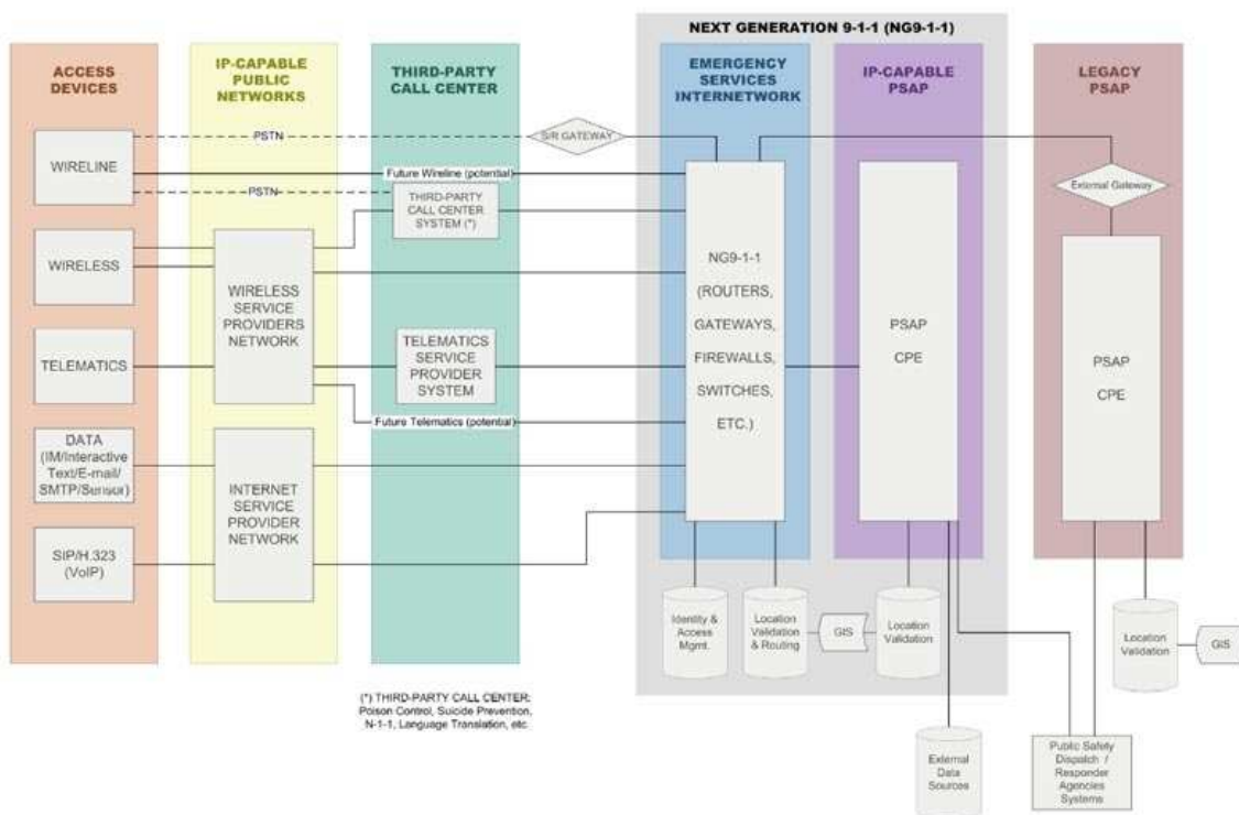
Obr. 26 Uspořádání systému NG911 (Boundary NG911) [80]
