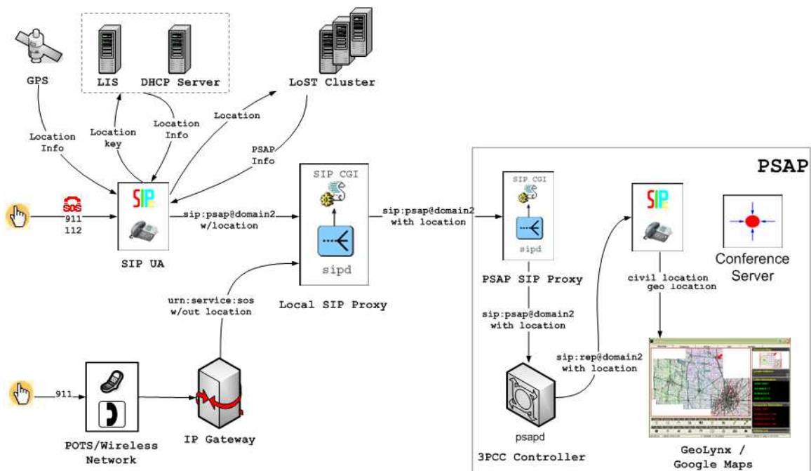
Obr. 29 Základní architektura Next Generation 911 [82]
