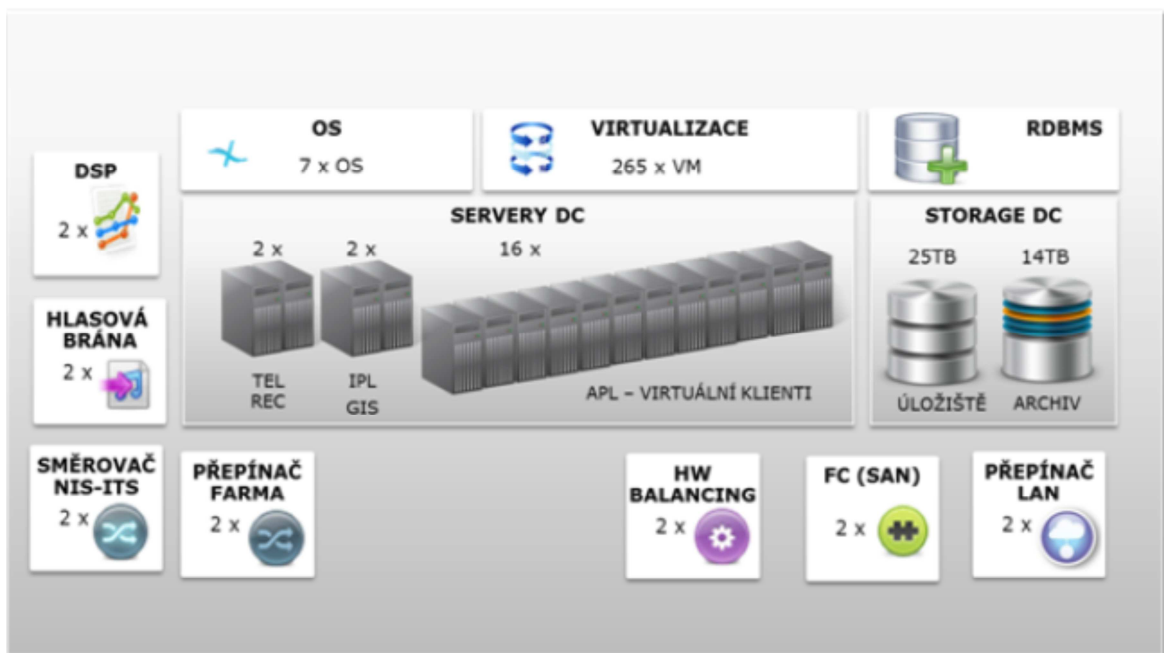
Obr. 16 Technické řešení datového centra projektu NIS IZS [56]
