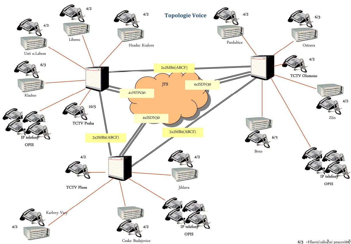
Obr. 9 Rozmístění a propojení TCTV 112 [37]
