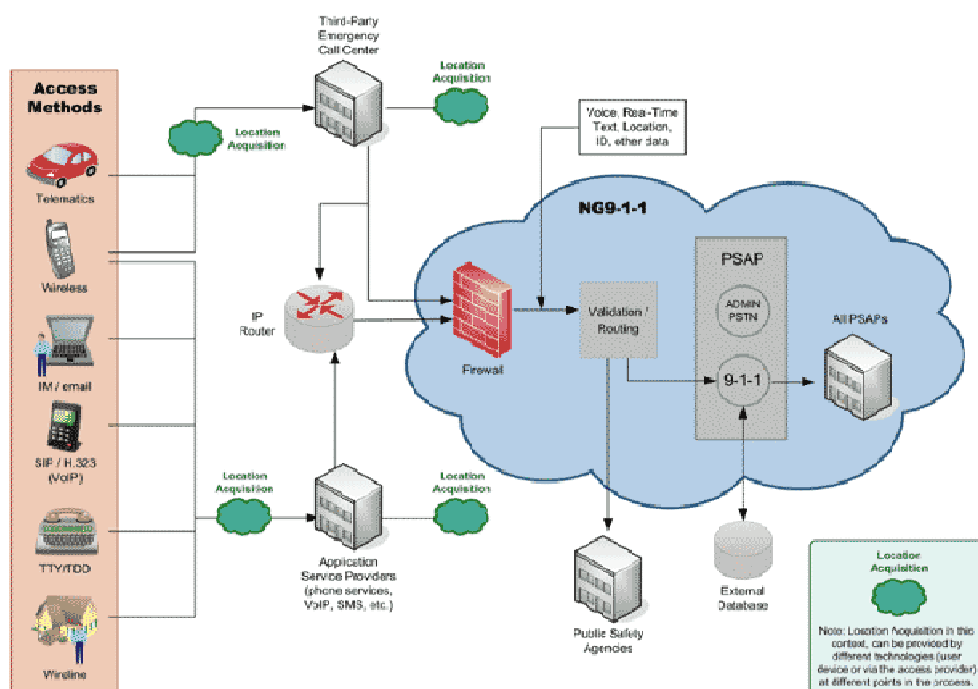
Obr. 28 Blokové schéma systému NG911 [80]
