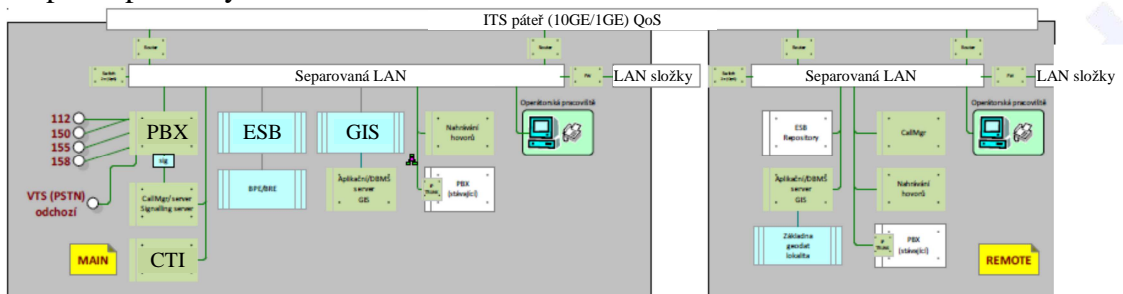
Obr. 19 Architektura NSPTV – IP telefonie [55]
