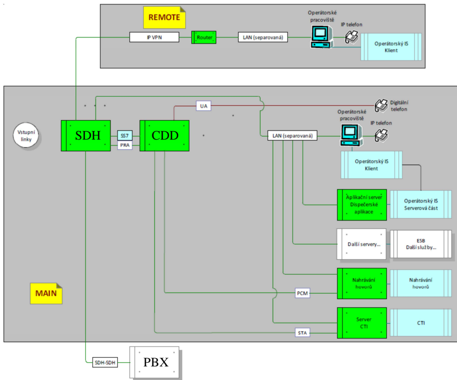
Obr. 18 Architektura NSPTV - kombinovaná duální telefonie [55]
